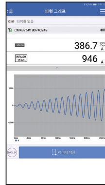
파형 그래프 간이 오실로스코프 (전압, 전류)
