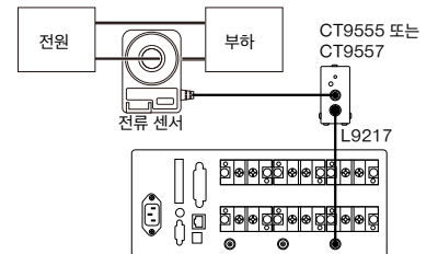
TYPE2 전류 센서 연결 이미지
