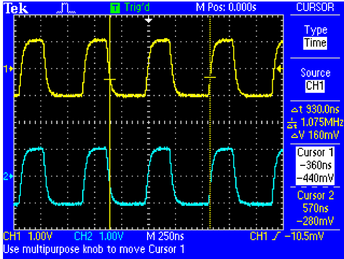
파형을 쉽고 빠르게 캡처
