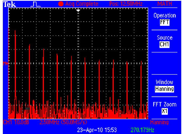
고급 연산 기능을 포함한 FFT의 신속한 실행 가능
