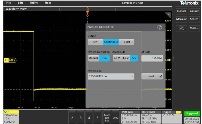
디지털 패턴 발생기
